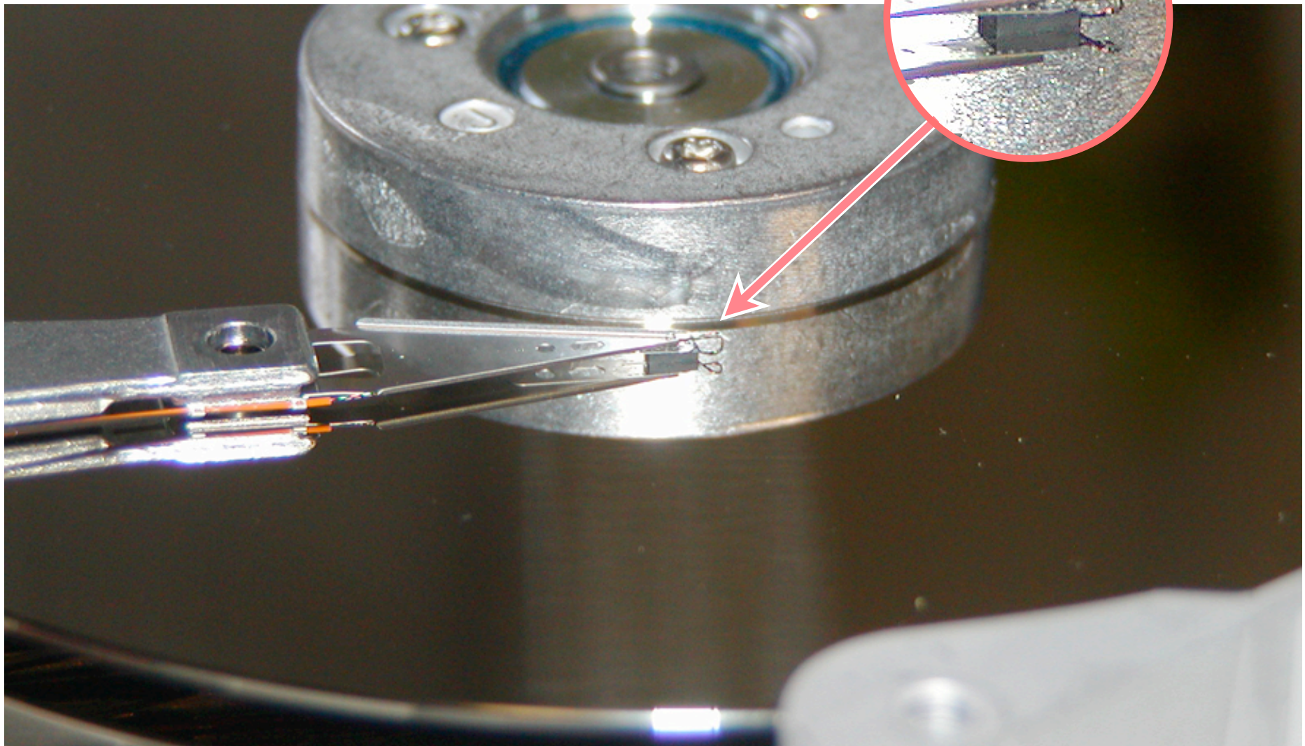
磁気ヘッド（スライダ）は 2mm x 1mm 以下程度の大きさ
